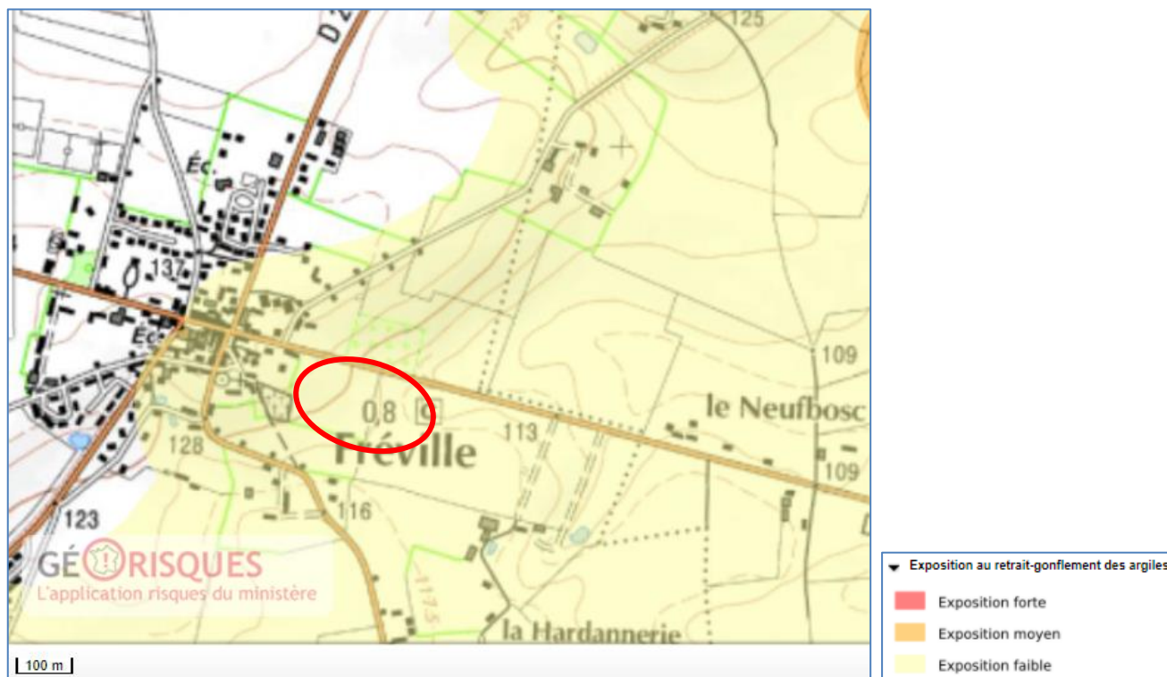
Carte d'exposition vis-à-vis du retrait-gonflement des argiles – Extrait du site http://www.georisques.gouv.fr
