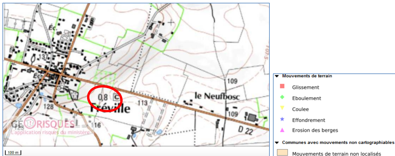
Carte d'aléa de mouvement de terrain – Extrait du site http://www.georisques.gouv.fr
