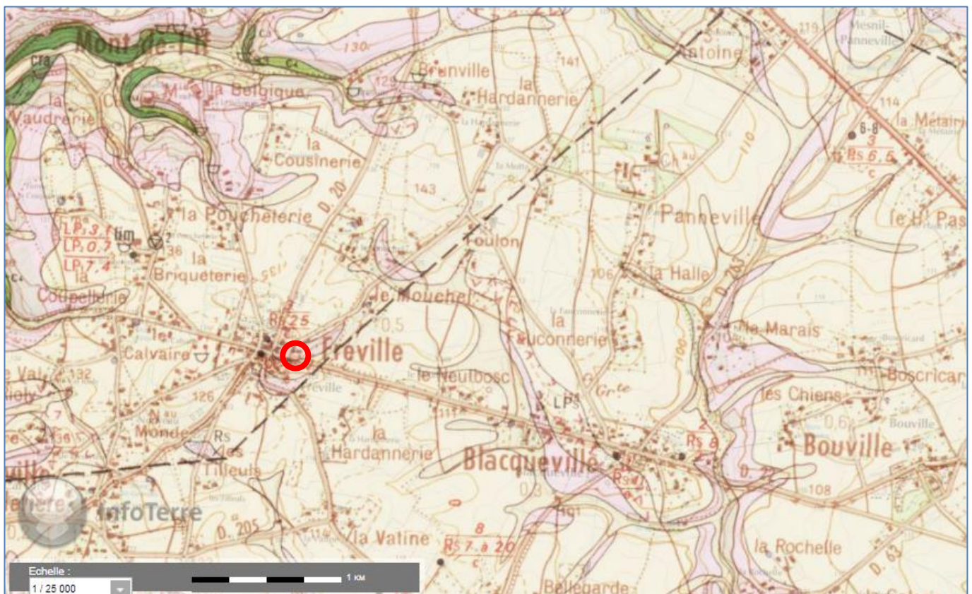
Extrait de la carte géologique d'YVETOT au 1/25000 ème , source https://infoterre.brgm.fr
