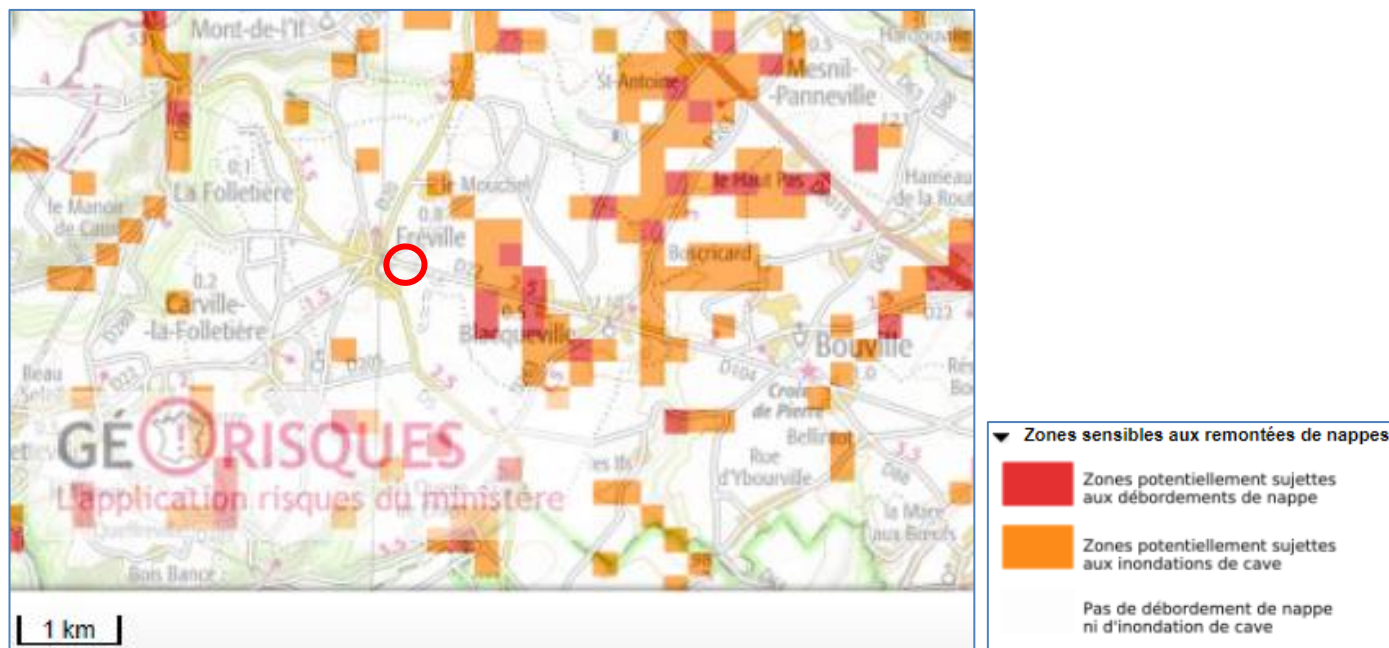
Carte du risque de remontées de nappes – Extrait du site https://www.georisques.gouv.fr
